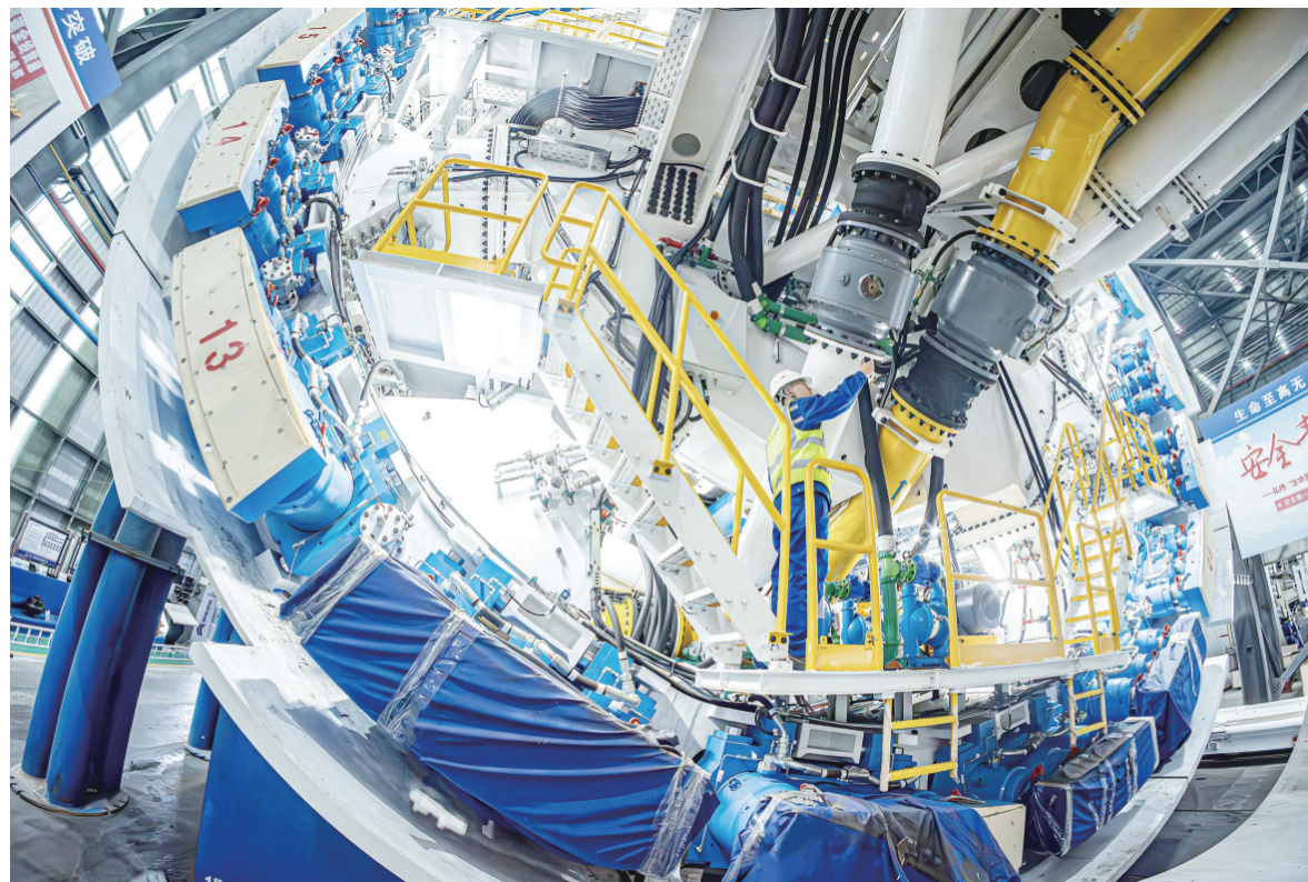
3月31日，中铁十四局监造人员验收盾构机泥浆环流系统。
